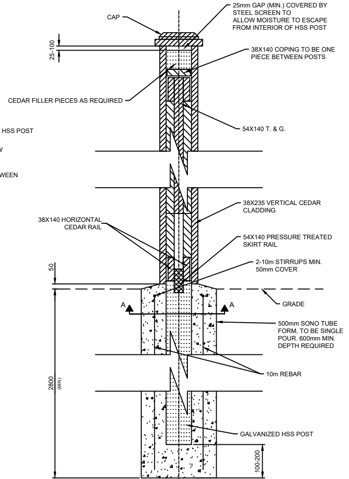
TYPICAL SECTION N.T.S.
