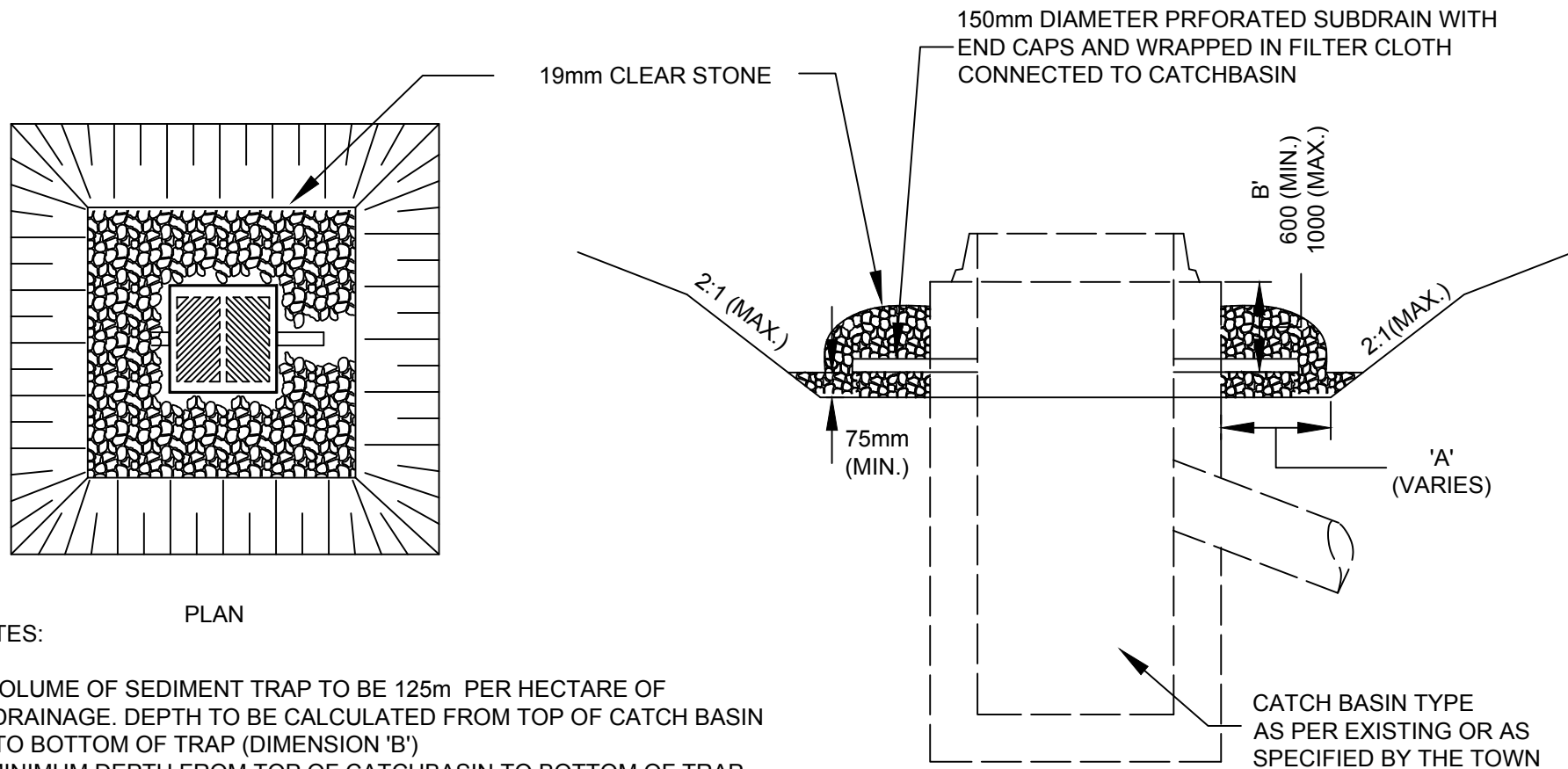
SECTION A-A
