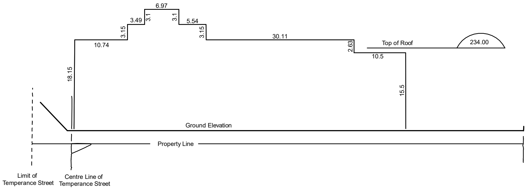
SECTION A-A
