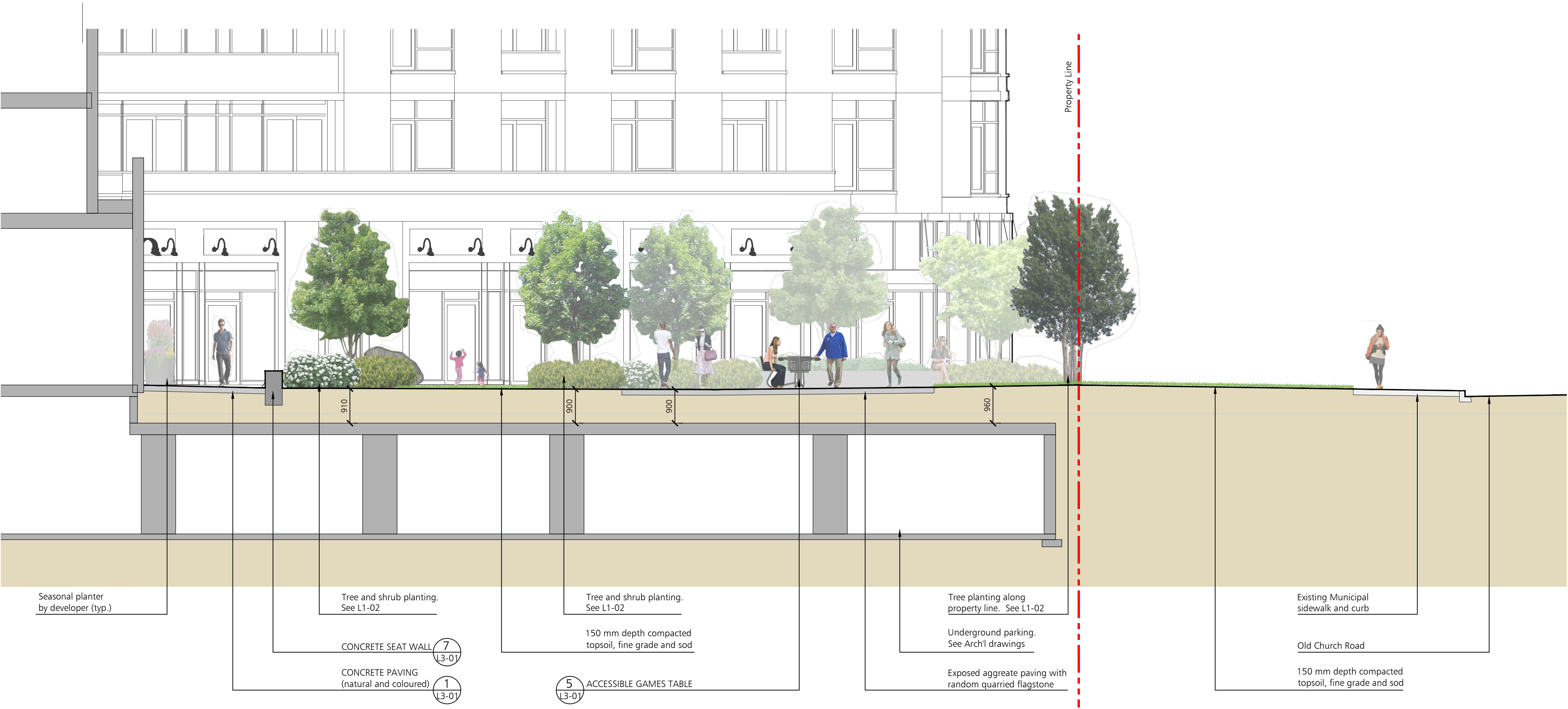
Section A - A' 1:750
