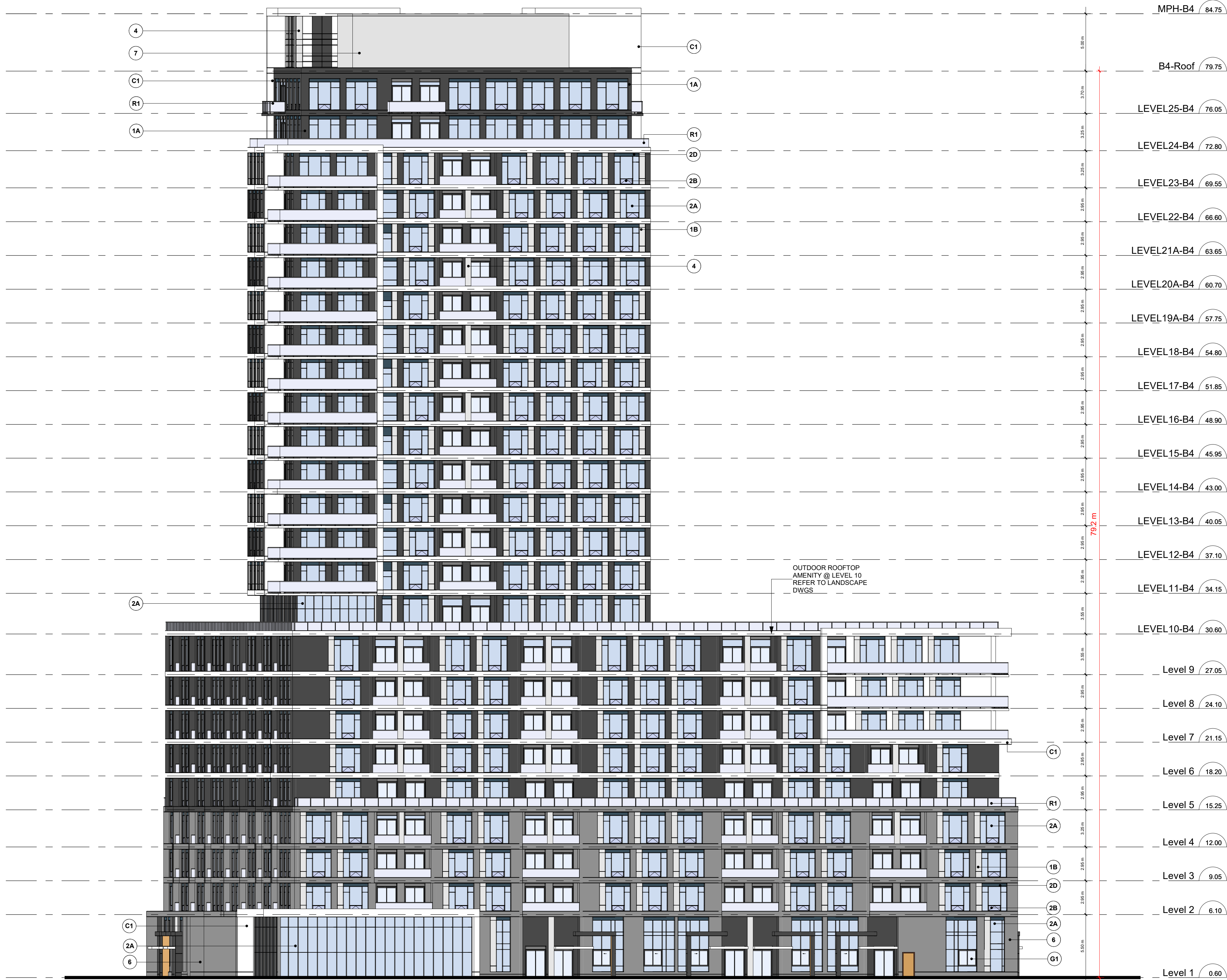
B4 WEST ELEVATION 1 Scale: 1 : 200 A419
