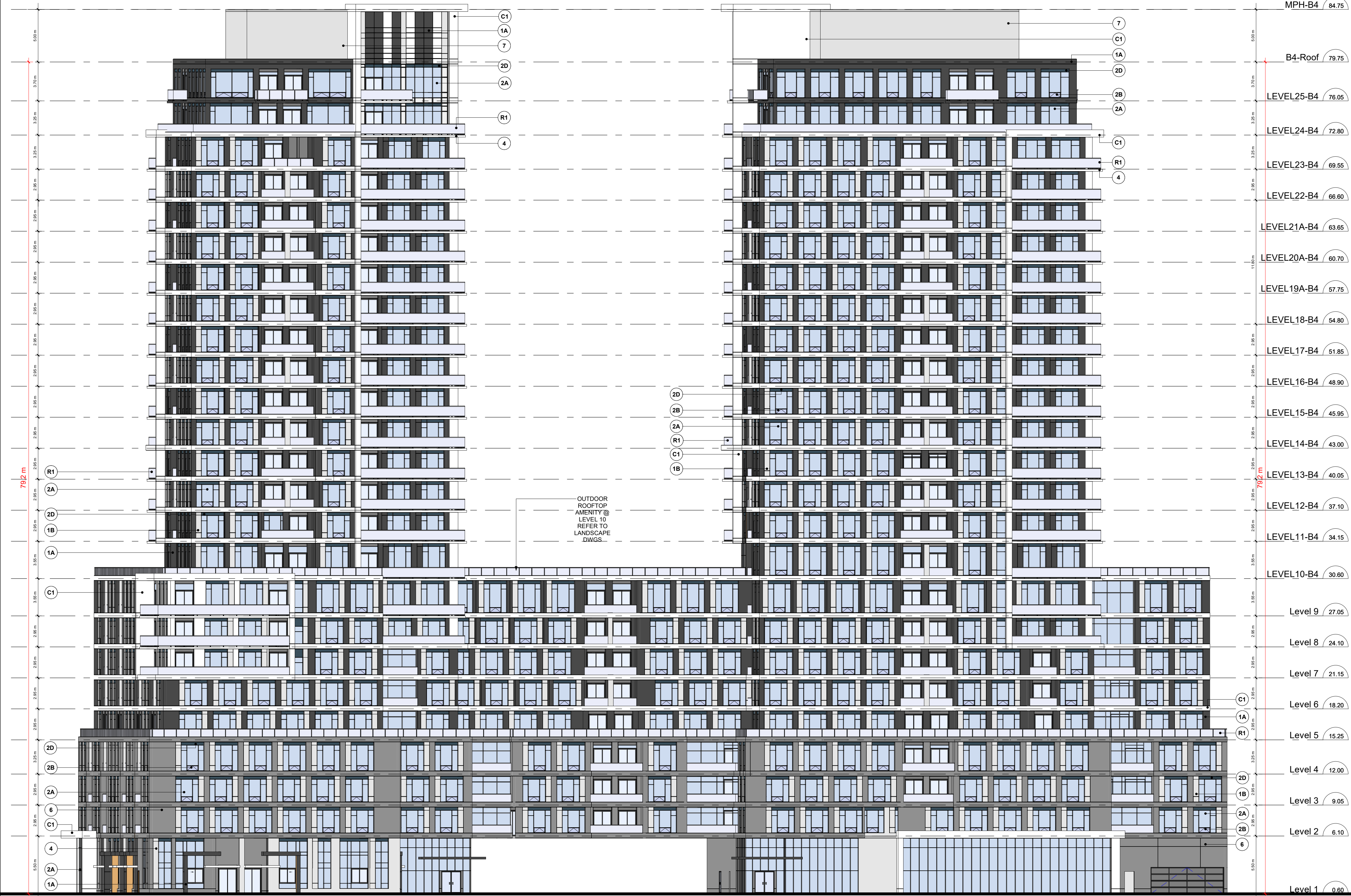
B4 SOUTH ELEVATION 1 Scale: 1 : 200 A418
