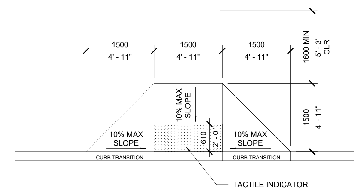
D1 CURB CUT SCALE: 1 : 50
